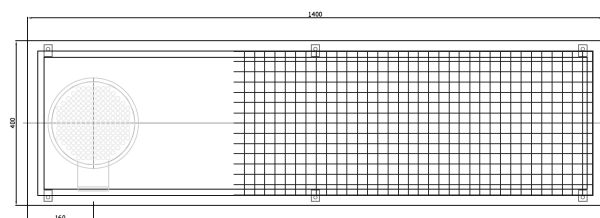
Alto
